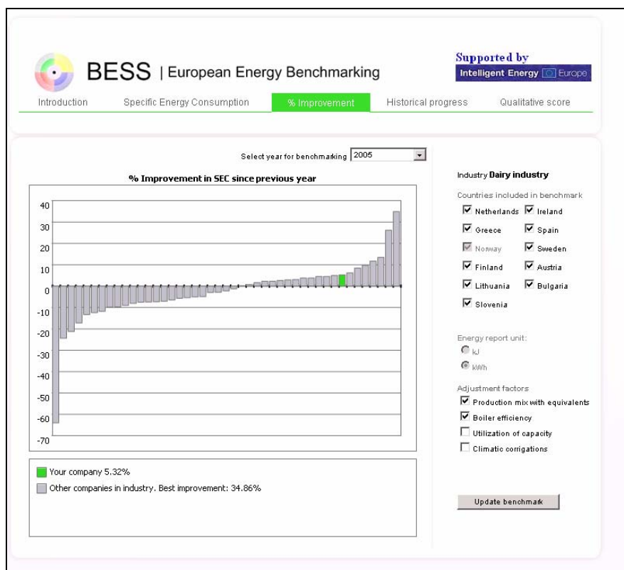
Diagramm 2: Entwicklung des spezifischen Energieverbrauchs (Unterschied zum letzten Jahr in Prozent).
