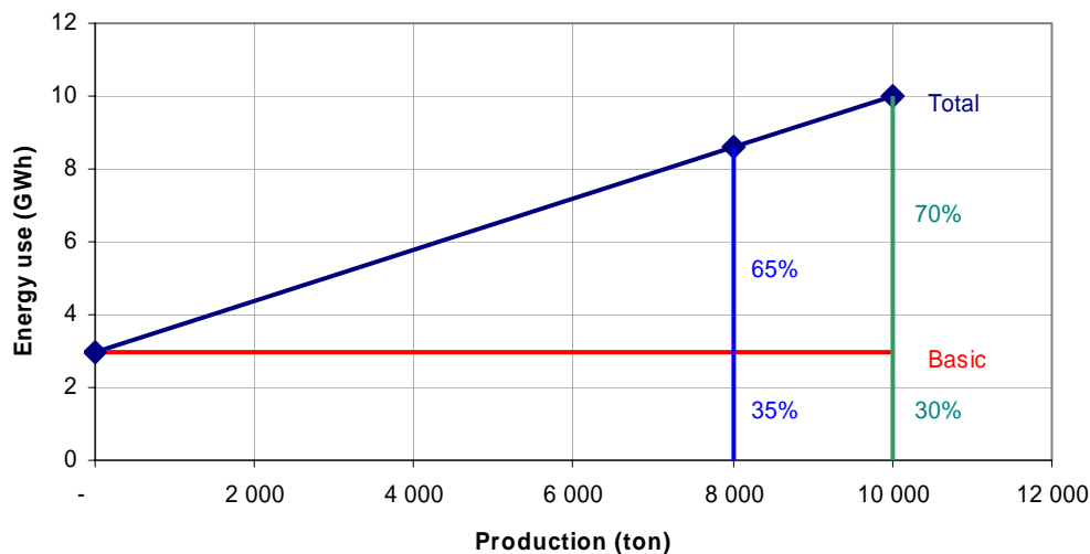
Abbildung 1: Der Anteil des Grundenergieverbrauchs steigt, wenn die Kapazitätsauslastung sinkt
